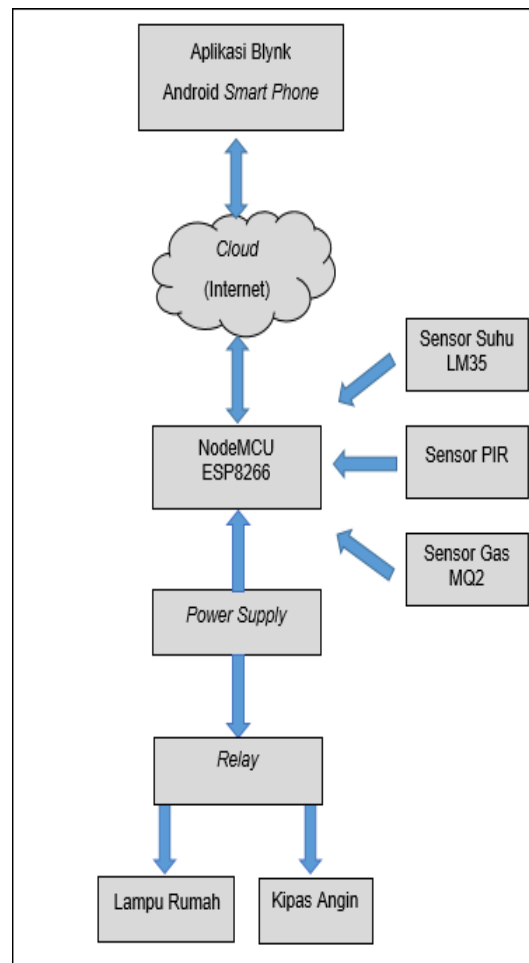
Gambar 1. Diagram Blok Perancangan sistem
